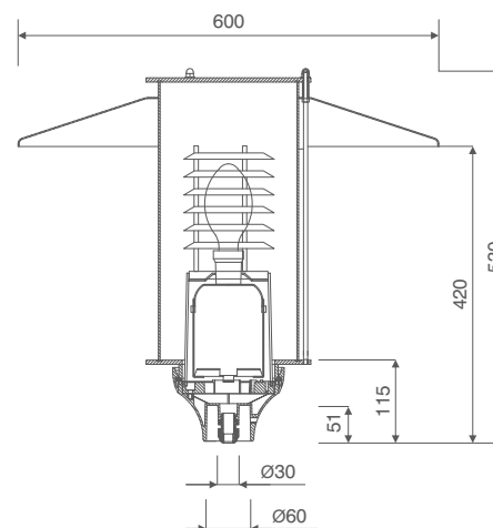
Oprawa ELBA z kloszem przezroczystym
