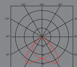
PISA IP65 PAR
