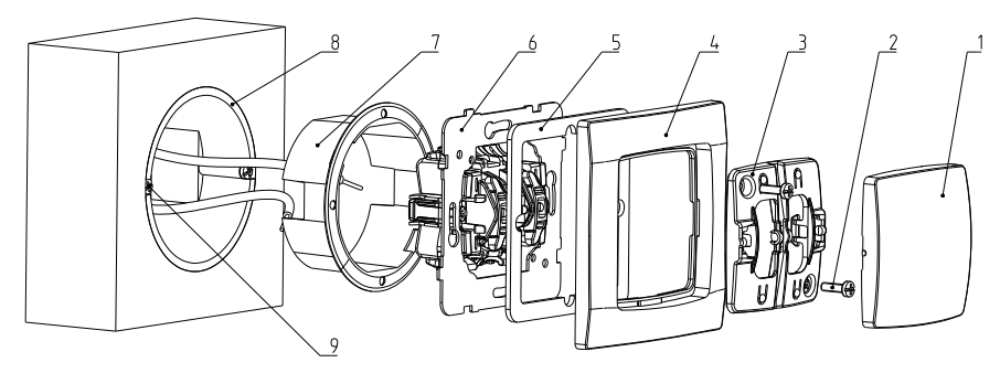
Rys.2/ Schemat instalacji łączników IP-44 serii Karo.
