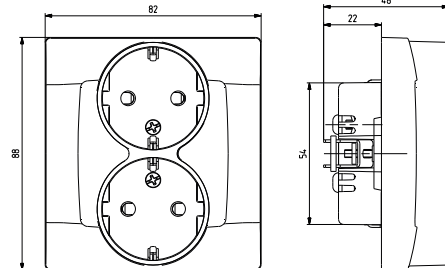
Gniazdo podwójne schuko
