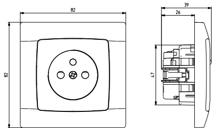
Gniazda pojedyncze IP-20
