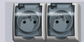
GNH-2HZ/00/d Gniazdo podwójne z uziemieniem 115
