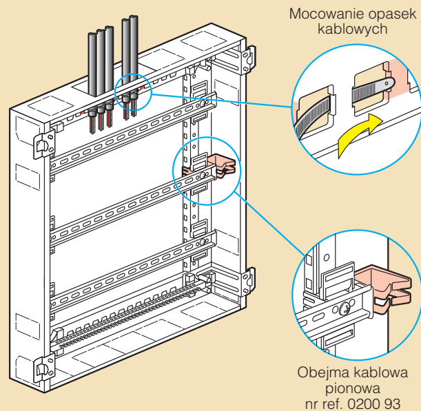
Demontowalna konstrukcja wsporcza
