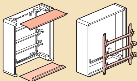
Demontowalne płyty górna i dolna
