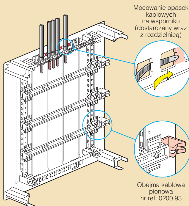
Demontowalna konstrukcja wsporcza
