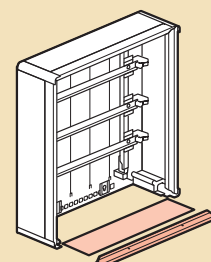
Demontowalne płyty górna i dolna
