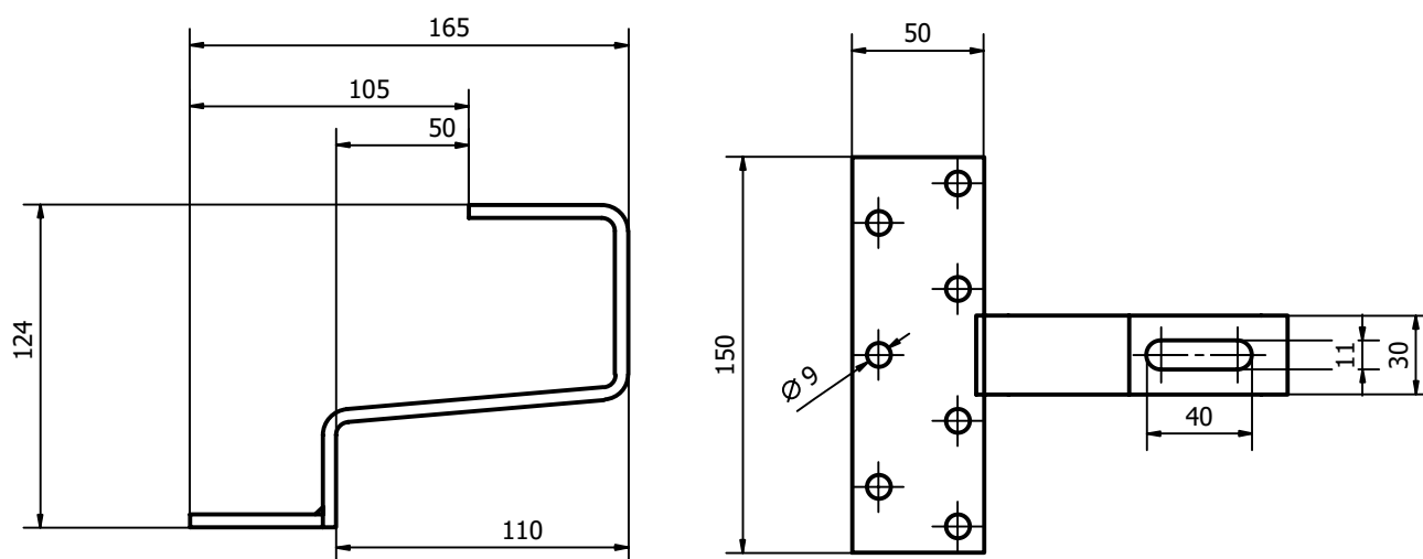
Rys.1 Wymiary elementu K-10
