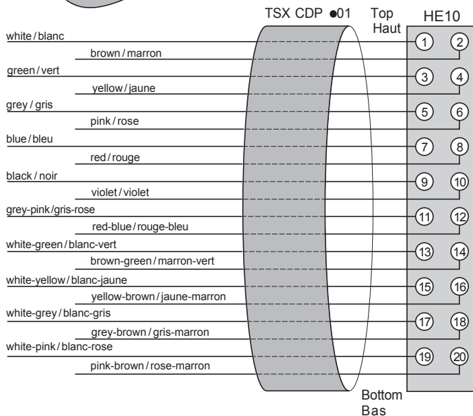
Prewired cable Toron précablé
