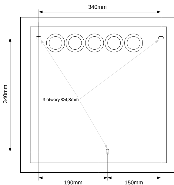
Rys. 7.1.1.1 Mocowanie centrali UCS w obudowie do 16A
