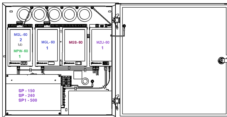
Rys. 1.1 Centrala UCS 6000 do 16 A
