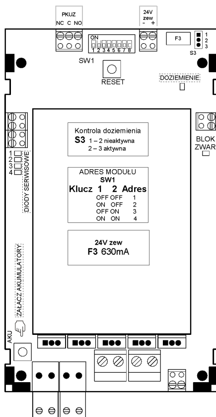
Rys. 4.7 Moduł MZU-60
