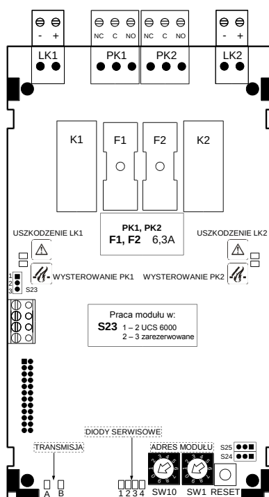
Rys. 4.4 Moduł MPW-60
