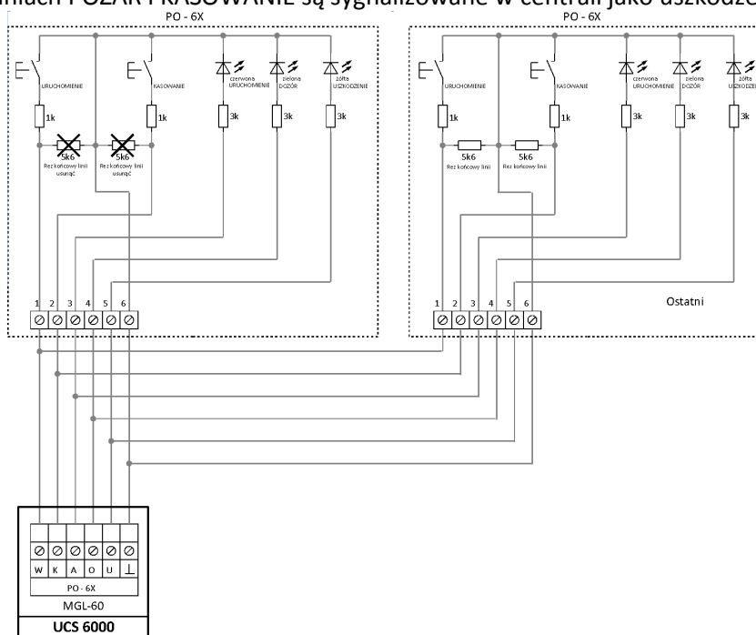
Rys. 4.3.2 Sposób podłączenia ręcznych przycisków oddymiania PO-6X do UCS 6000
