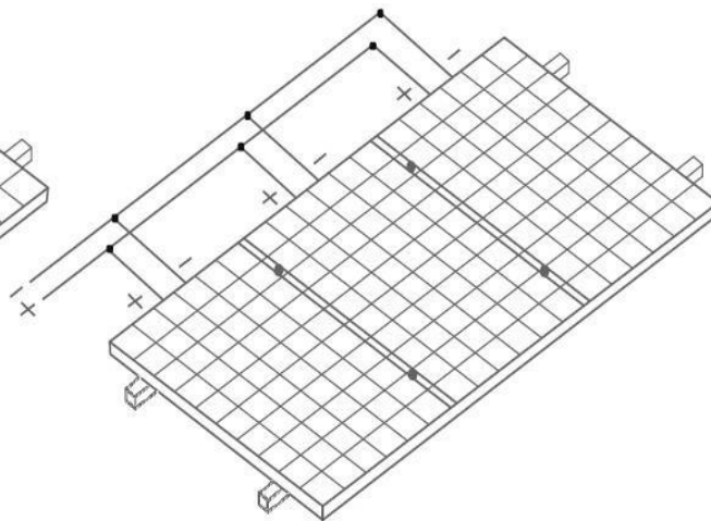
Rys.5 Połączenie równoległe
