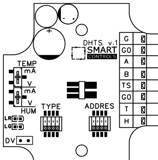
Rys.2. Wnętrze przetwornika
