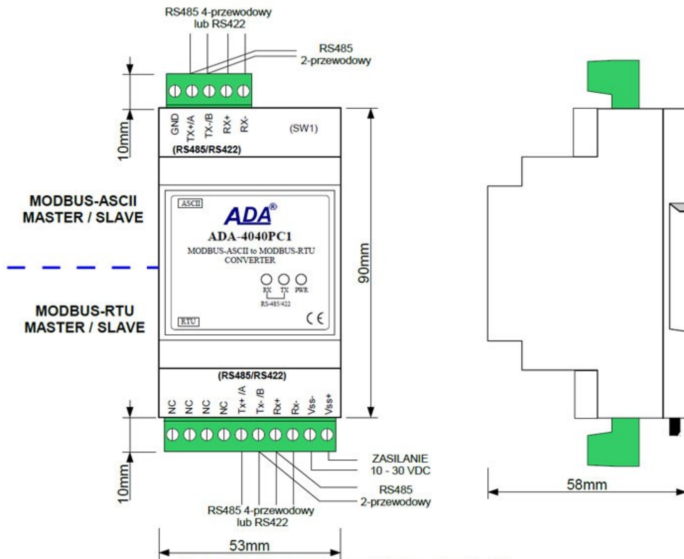
Rys 1. Widok ADA-4040PC1 oraz położenie przełącznika SW1
