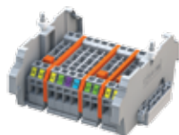
listwa pomiarowa ze zwieraniem torów prądowych za pomocą mostków
