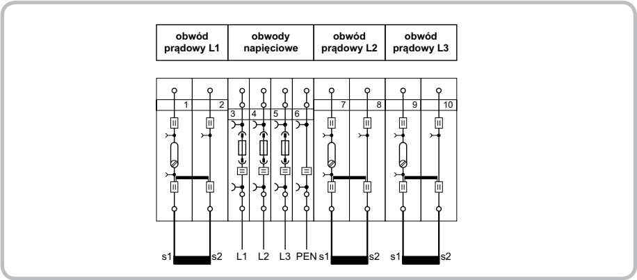
Schemat wewnętrzny listwy 847-767
