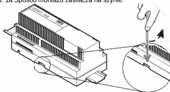
Rys. 1b Sposób montażu zasilacza na szynie.
